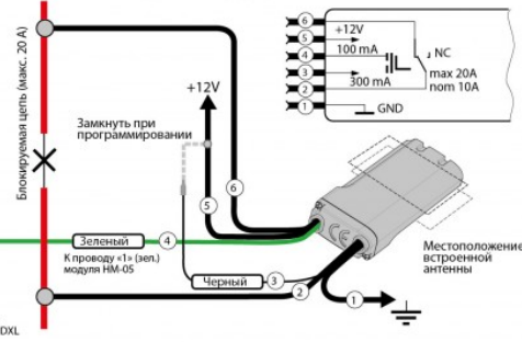
Схема подключения радиореле Pandect IS-119
