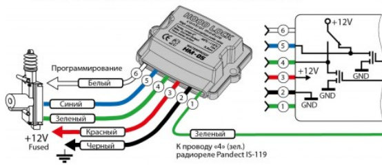
Схема подключения модуля управления замком капота NM-05
